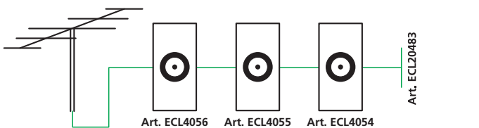
IMPIANTO TV CON DISTRIBUZIONE A CASCATA TV SYSTEM WITH FALL DISTRIBUTION Singolo utente / One user
