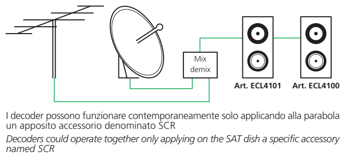
IMPIANTO TV CON DISTRIBUZIONE A CASCATA TV SYSTEM WITH FALL DISTRIBUTION Singolo utente / One user
